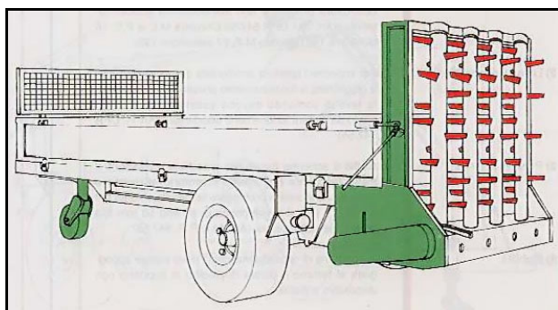
CARRO SPANDILETAME POSTERIORE PROVVISTO DI PROTEZIONI AGLI ORGANI DI TRASMISSIONE DEL MOTO
